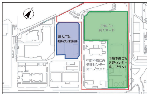
工事前の施設の設置状況
