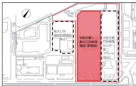
工事後の施設の設置状況
