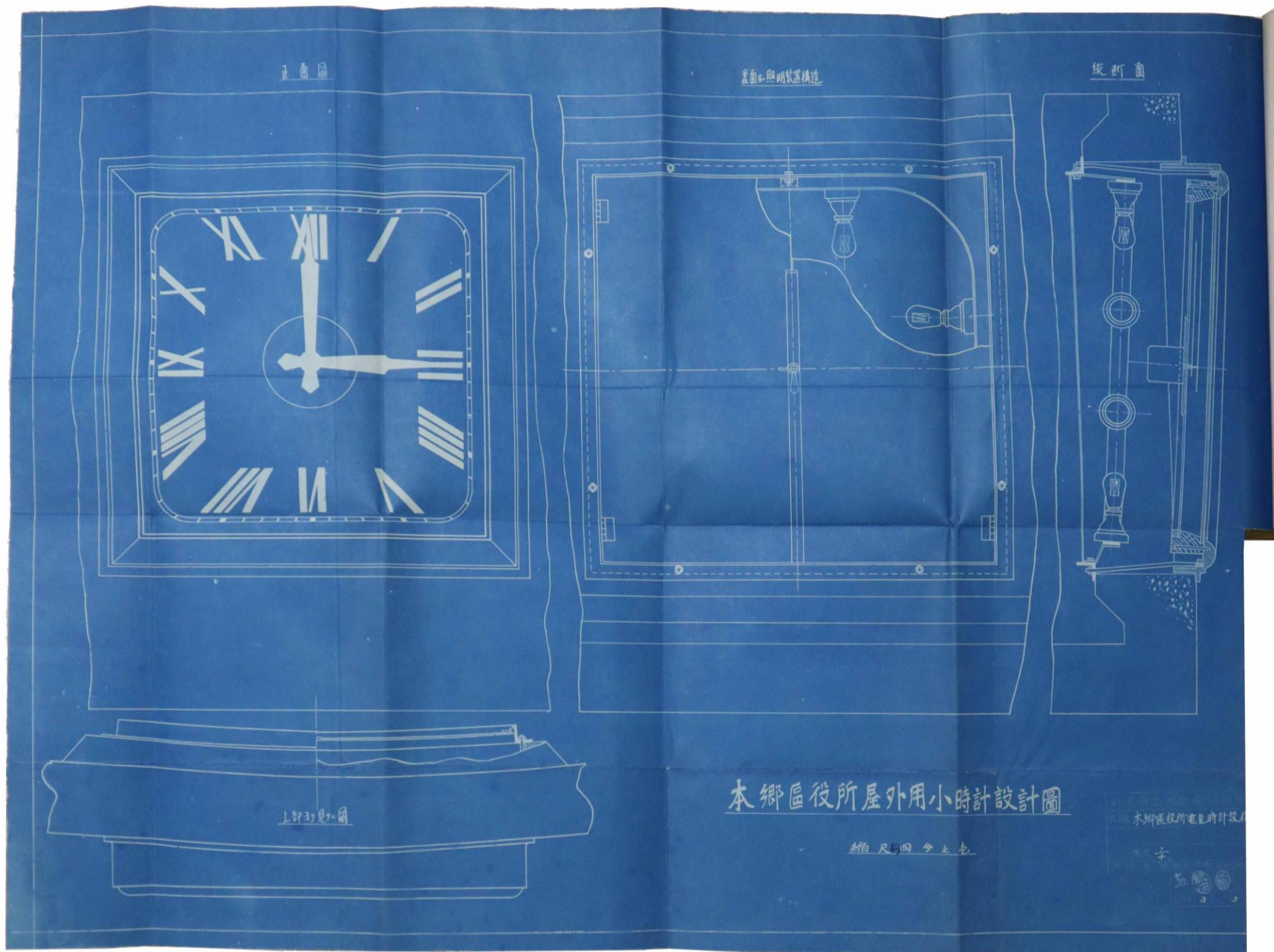
本郷区役所屋外用小時計設計圖
